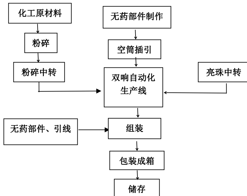
图 2-4-4 升空类（双响炮）生产流程图
