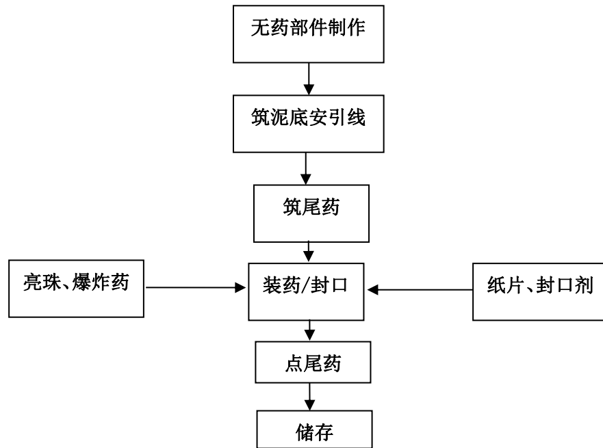
图 2-4-2 效果内筒生产流程图
