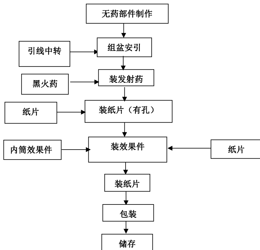
图 2-4-3 组合烟花产品生产工艺流程图
