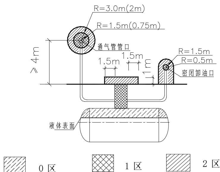
图3-4-1 埋地卧式汽油储罐爆炸危险区域划分
