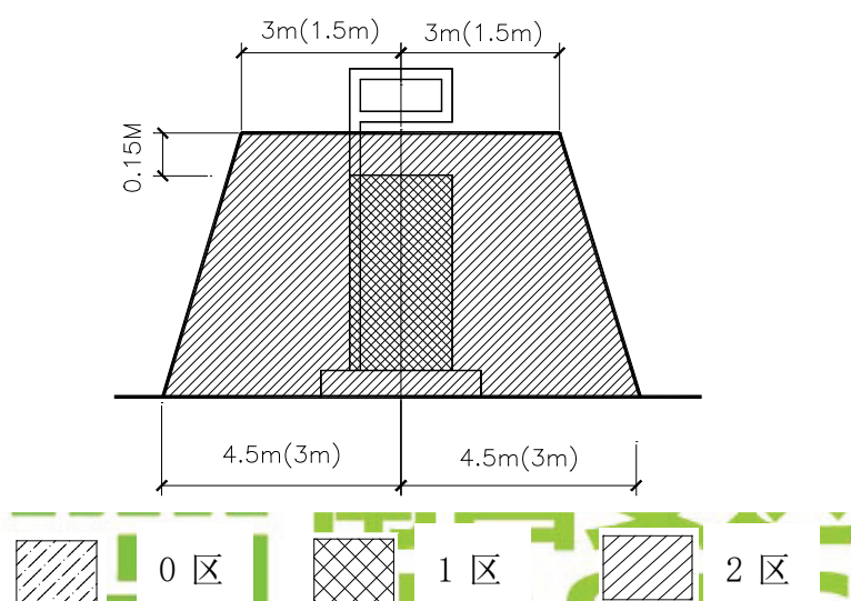
图 F3.3-2 汽油加油机爆炸危险区域划分
